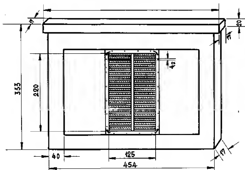
Преградна даска са Ханмановом решетком (Мере изражене у mm)
